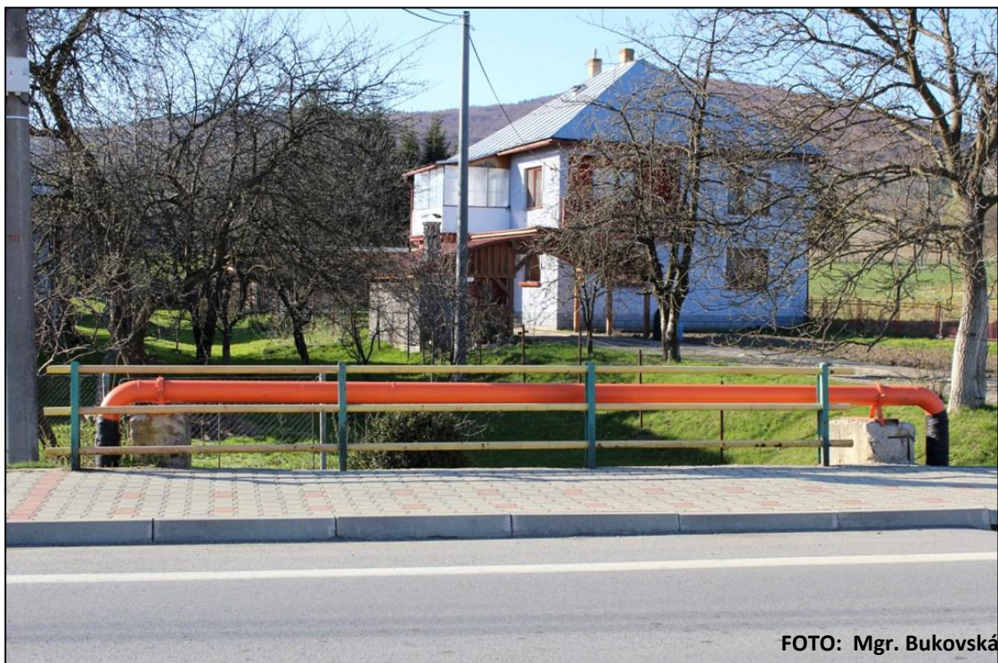
Obr. 3 – Križovanie plynového potrubia s mostom pri hlavnej ceste
