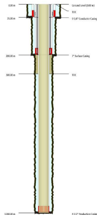
Konstrukce vrtu
